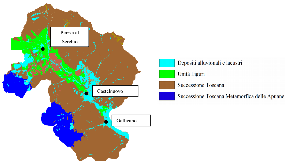
Distribuzione delle principali Unità Geologiche nel territorio dell'Unione dei Comuni
